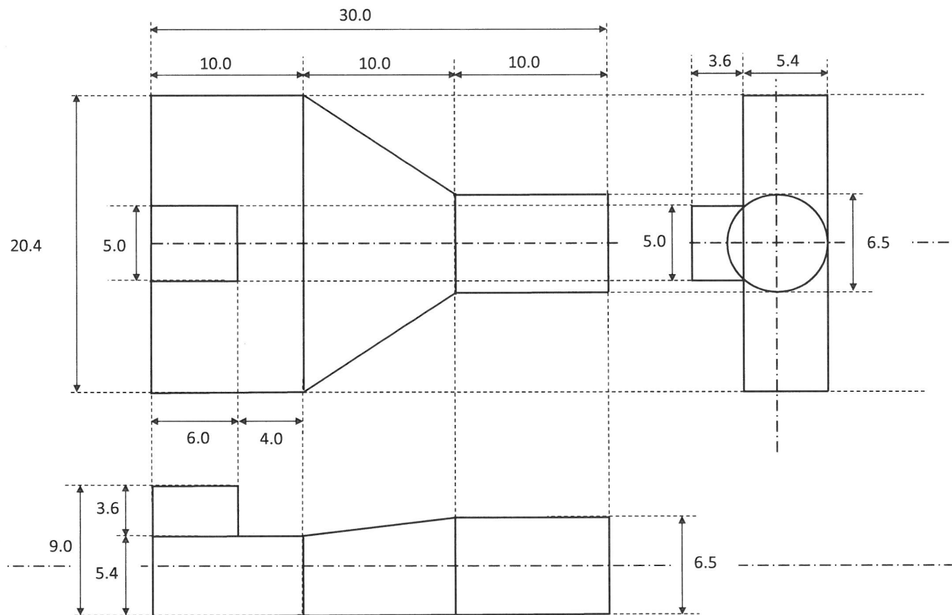
SMR-08V-NC用カバー (単位/mm) (08SMR-065)
